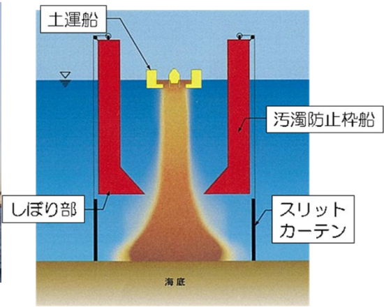
図-1 汚濁防止档概要
