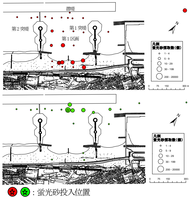
図-1 蛍光砂追跡調査
