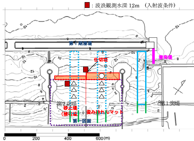
図-3 侵食対策工実証試験施設配置平面図
