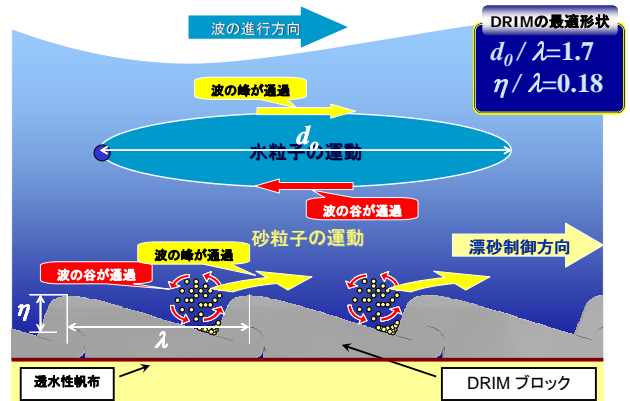
図-2 歪み砂れんマットの漂砂制御原理
