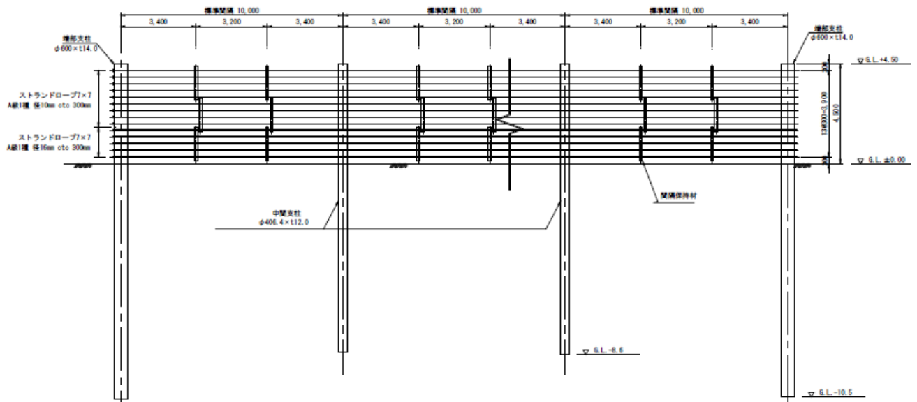
図-1 津波バリアーの試設計例
