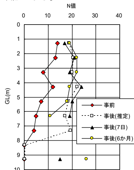
図-1 エコガイアストンの 改良前後の杭間 N 値
