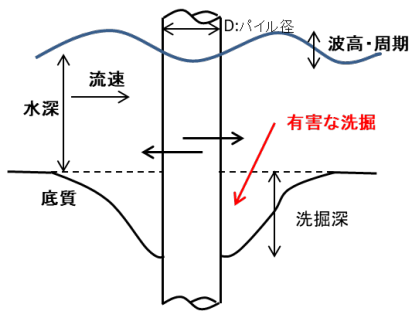
図-3 洗掘の要因
