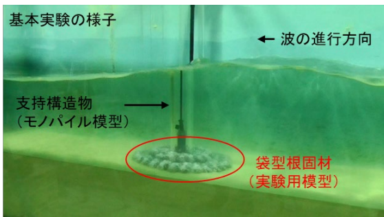
図-5 小規模実験の様子
