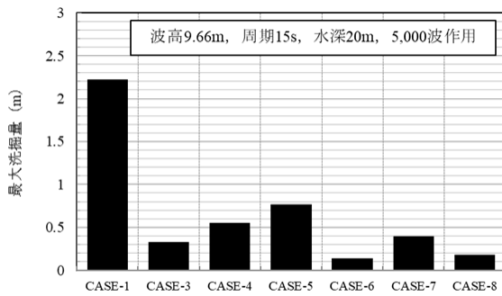
図-8 小規模実験での現地換算量としての最大洗掘量
