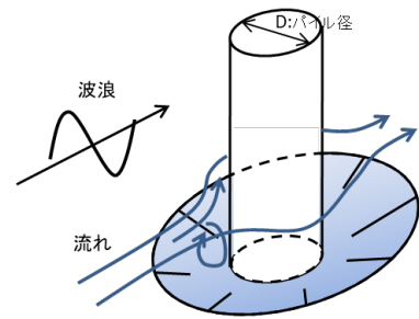
図-1 洋上風力発電設備への洗掘の影響
