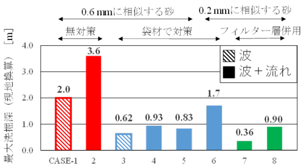
図-11 大規模実験での現地換算量としての最大洗掘量
