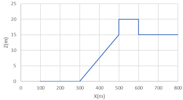
図 2.2-1 地形データの例 (X, Z 成分)
